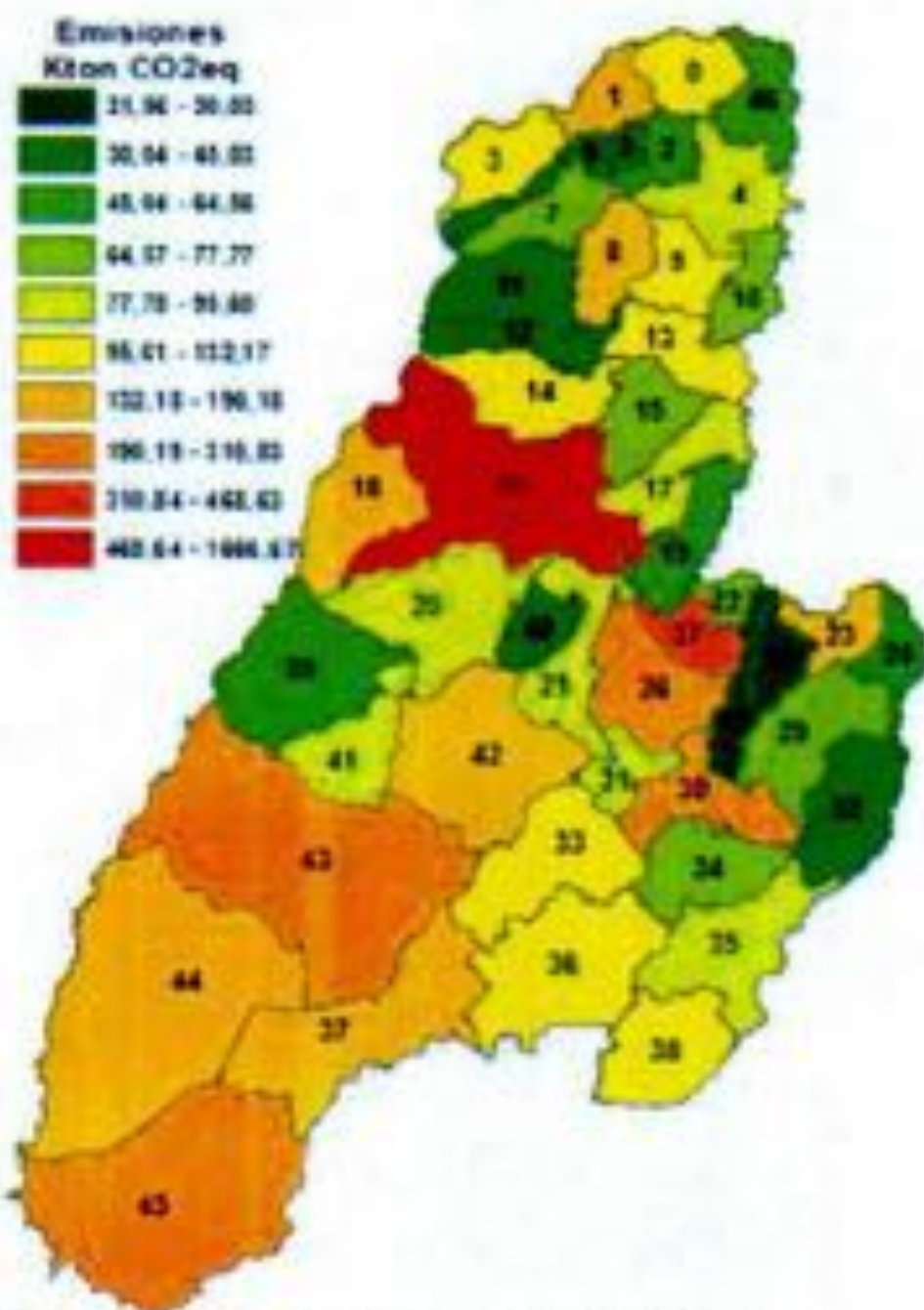
Ilustración 13 Mapa Emisiones en Kton CO 2 eq por municipios
