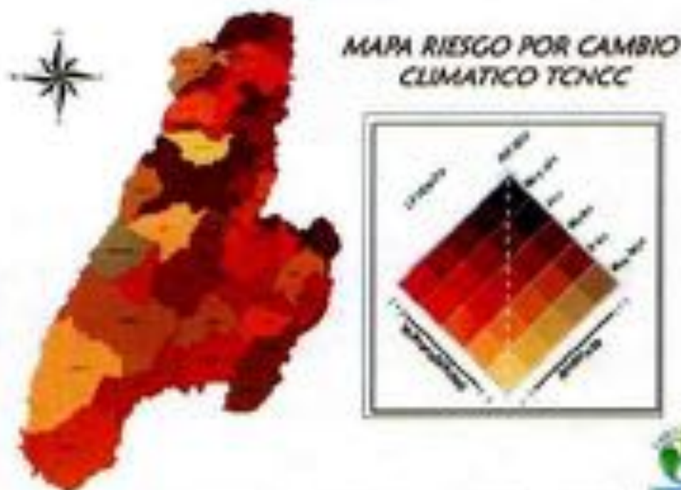
Figura 14 Mapa Riesgo por Cambio Climático TCNCC
