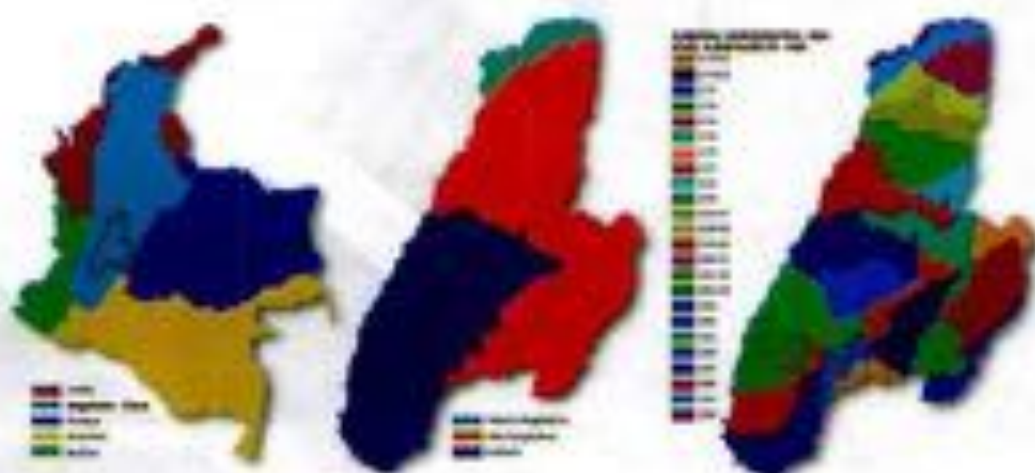
Ilustración 2 Mapa Zonificación-Hidrográfica Departamento del Tolima
