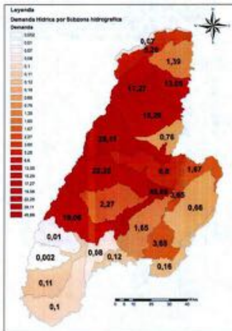
Mapa de distribución de la Demanda Hídrica en m3/seg por Subzona Hidrográfica
